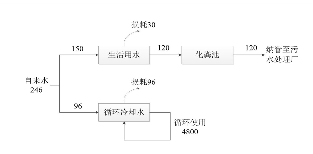
图 2-1 全厂水平衡图 (t/a)
