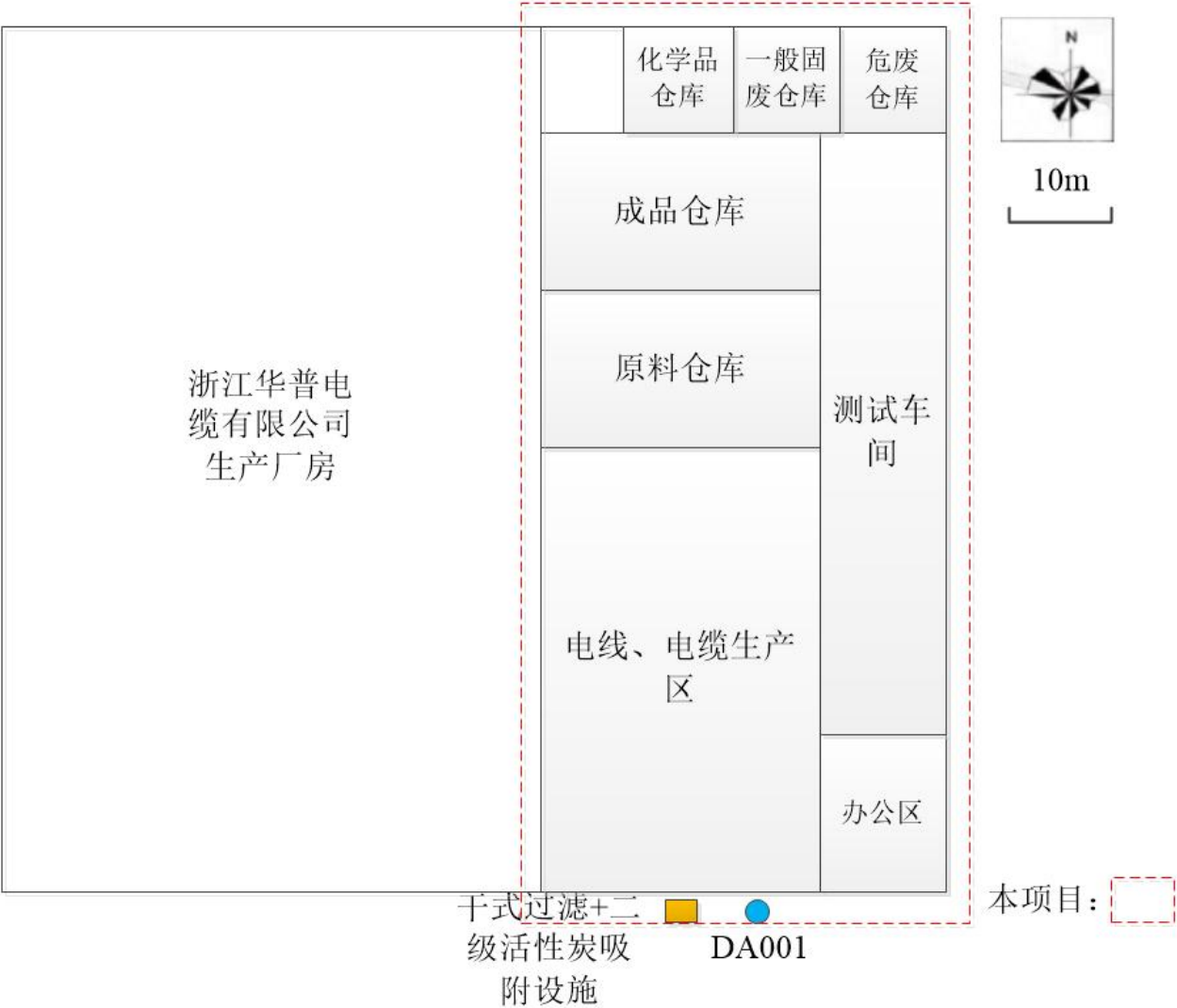
附图 5 建设项目厂区平面布置图
