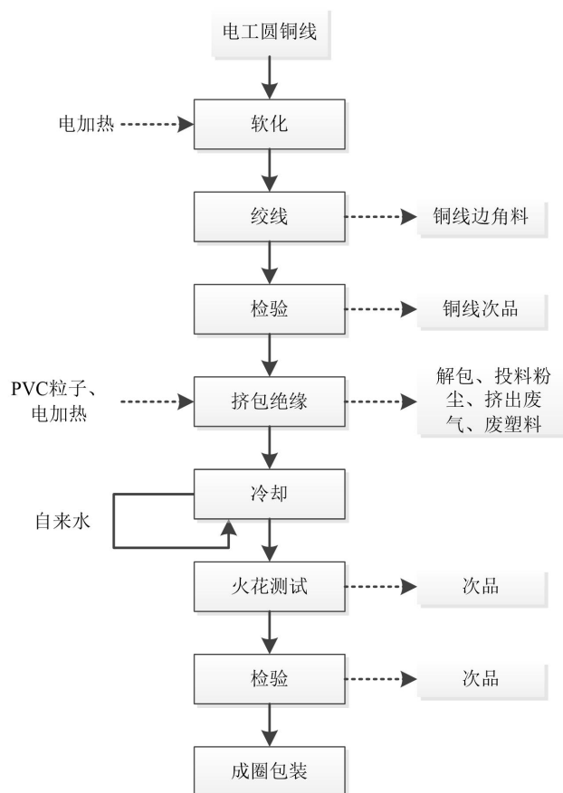
图 2-3 电线生产工艺流程图
