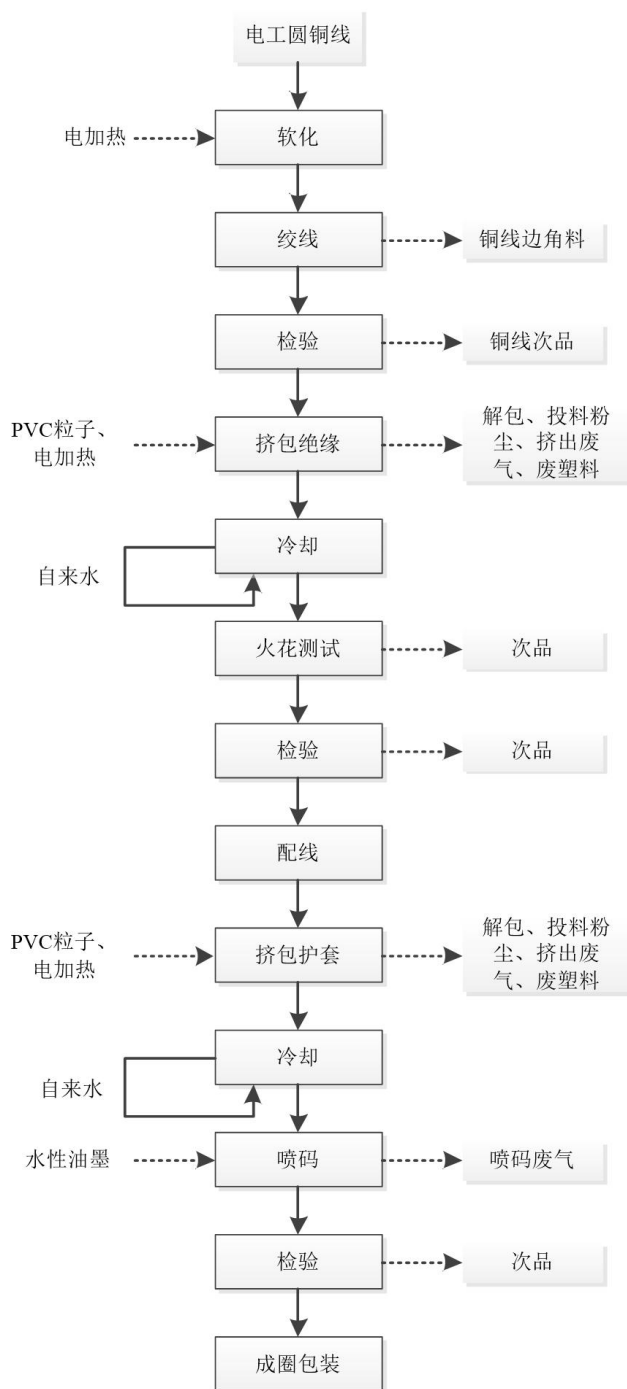
图 2-4 电缆生产工艺流程图
