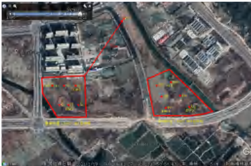
图 4.1-1 监测点位布置图
